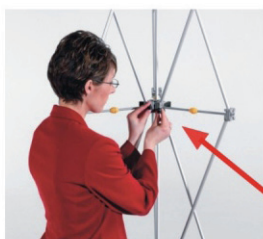
Ouvrez les 3 cotés de la structure fixer les cotés ensemble avec les magnétiques correspondants.
